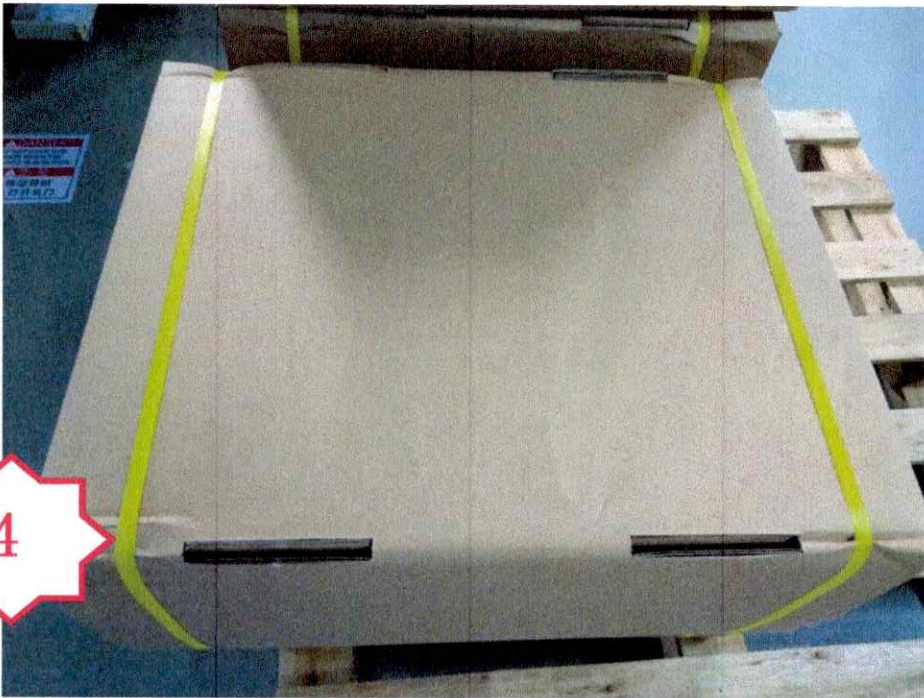
图四, 确认 PA02303 无漏装后, 将 22 的内箱与外箱配合并打包装带待出货
